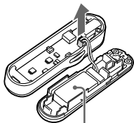
Batería recargable
